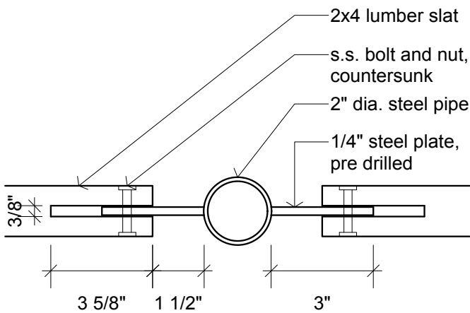
Plan Detail Scale: 3" = 1'-0"
