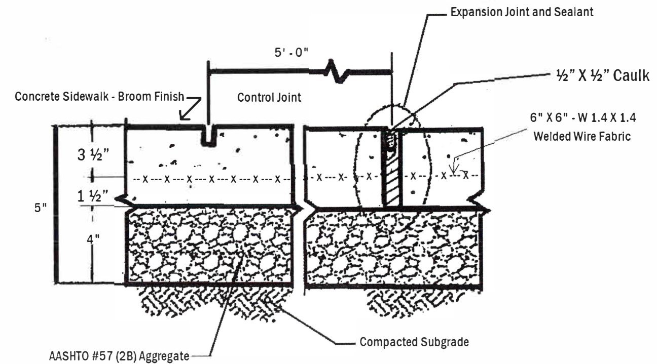
SIDEWALK DETAIL N.T.S.
