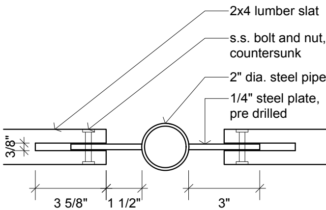
3 Plan Detail Scale: 3" = 1'-0"
