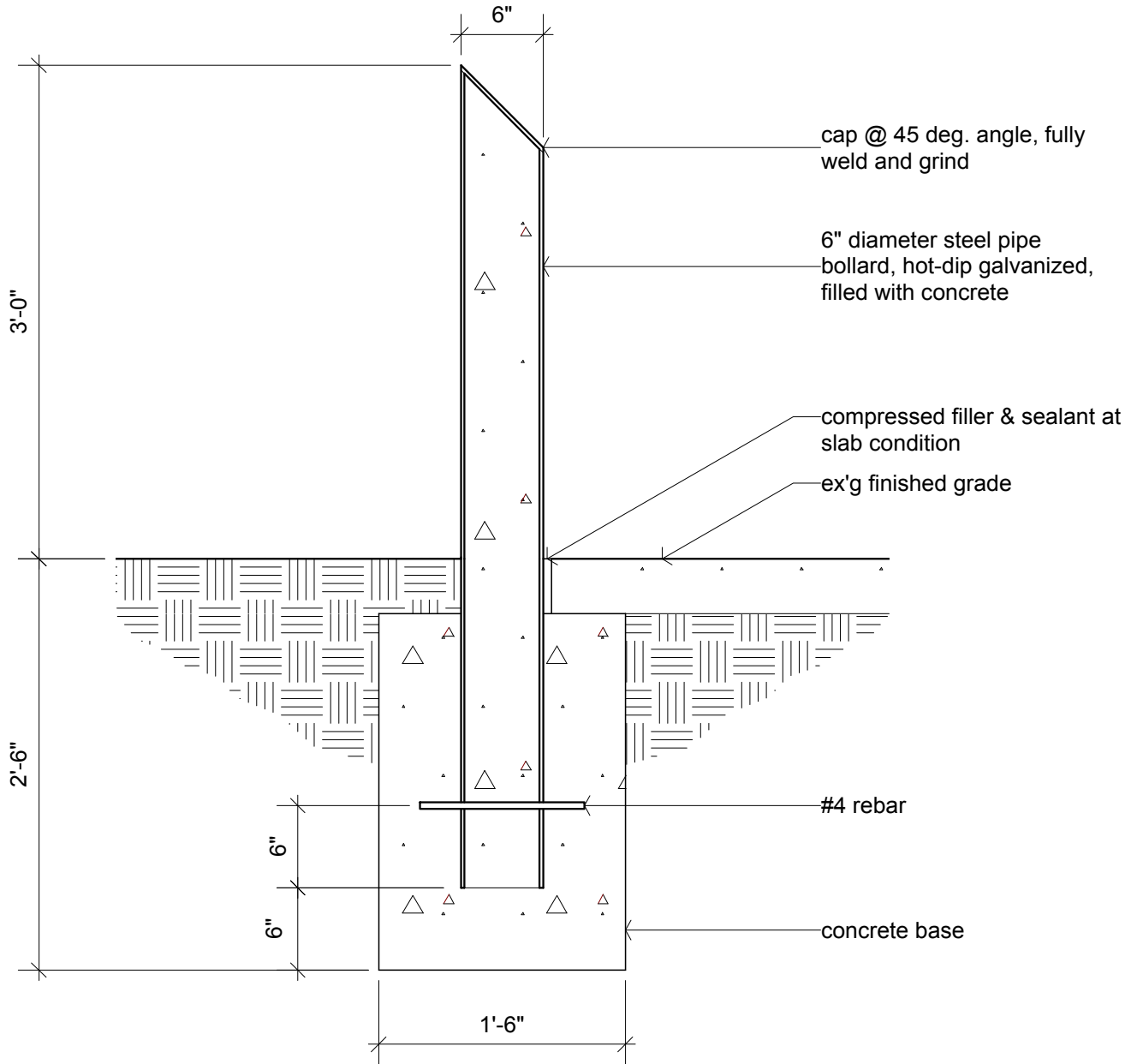
2 Steel Pipe Bollard Scale: 1" = 1'-0"
