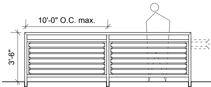
2 Guard Elevation Scale: 1/4" = 1'-0"
