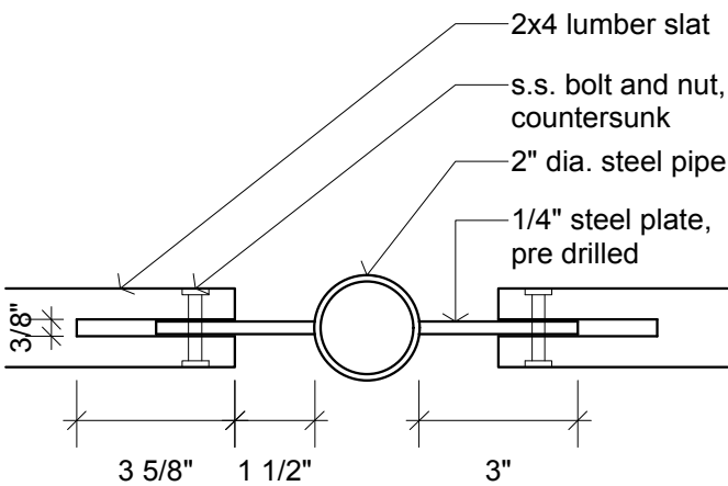
3 Plan Detail Scale: 3" = 1'-0"
